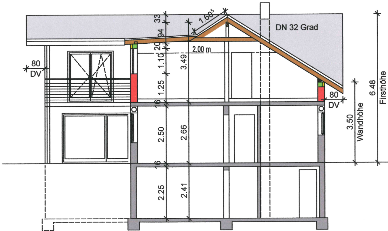
Schnitt 1-1
