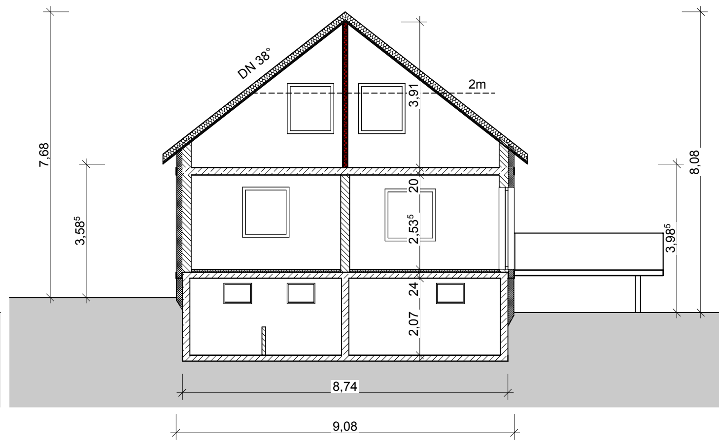
Schnitt 2
