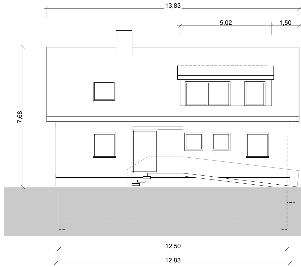
Ansicht Nord
