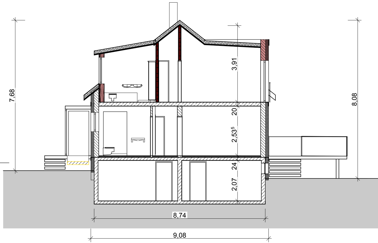
Schnitt 1
