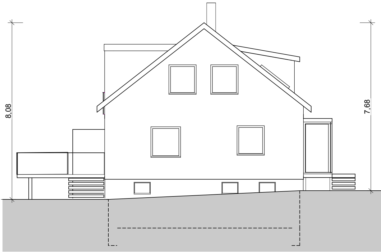
Ansicht Ost
