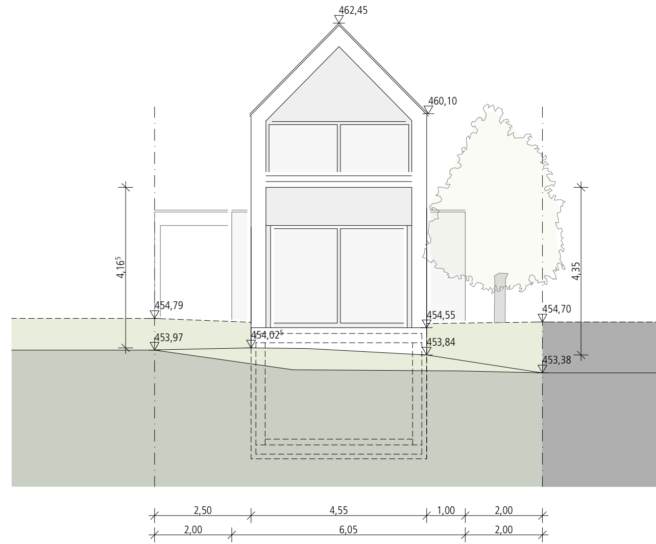
Ansicht Süd
