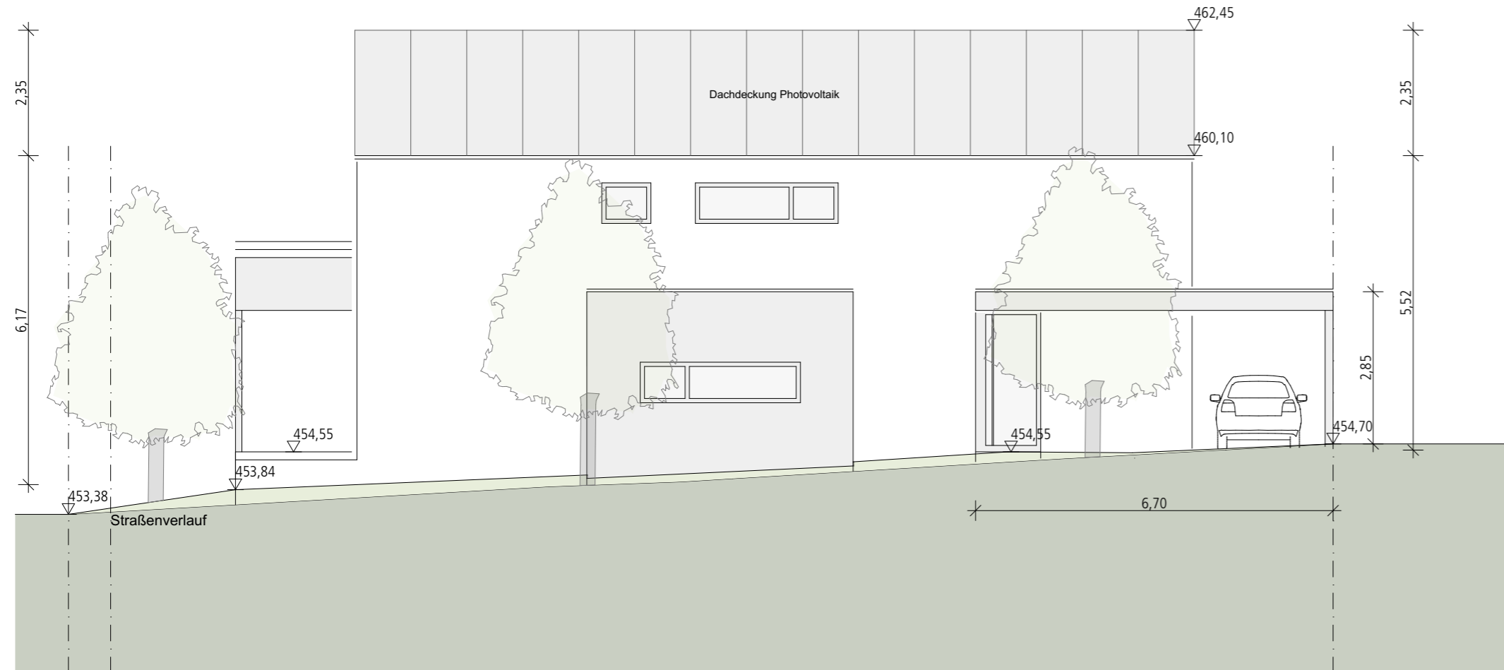
Ansicht Ost
