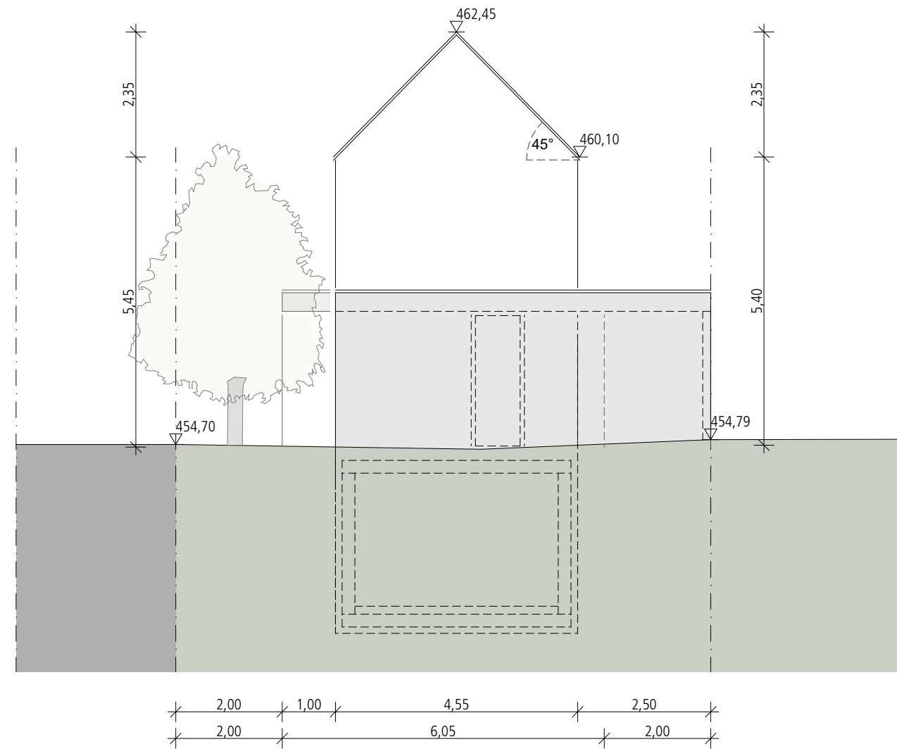
Ansicht Nord
