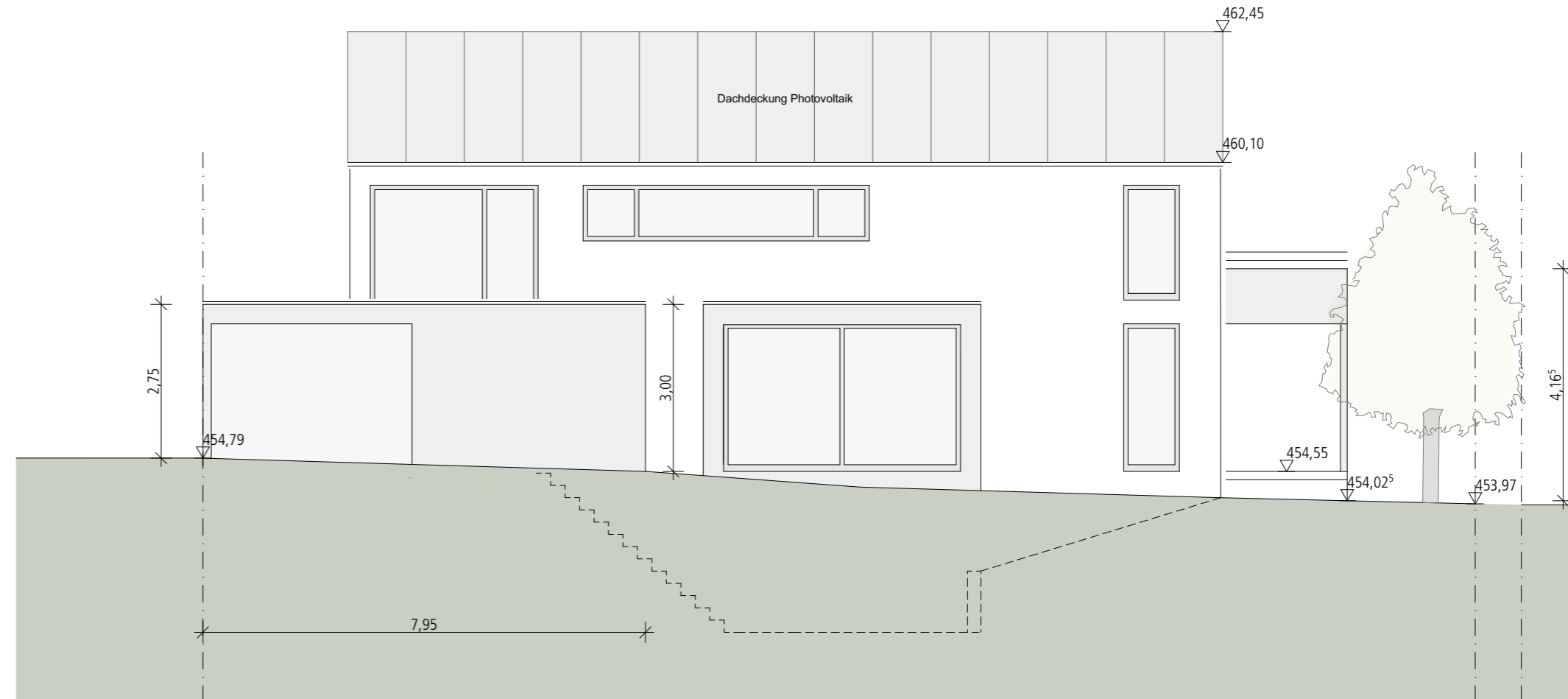
Ansicht West
