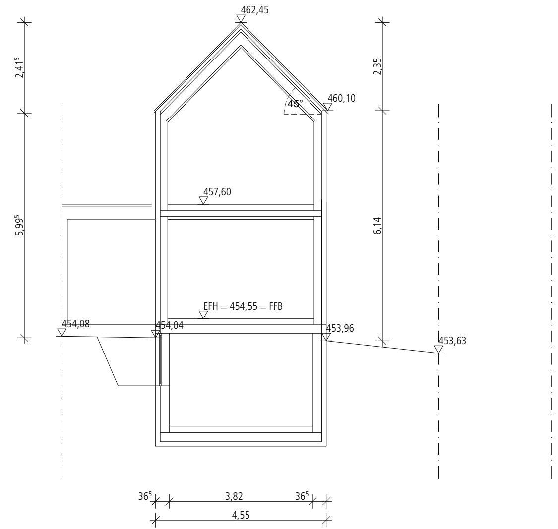
Querschnitt
