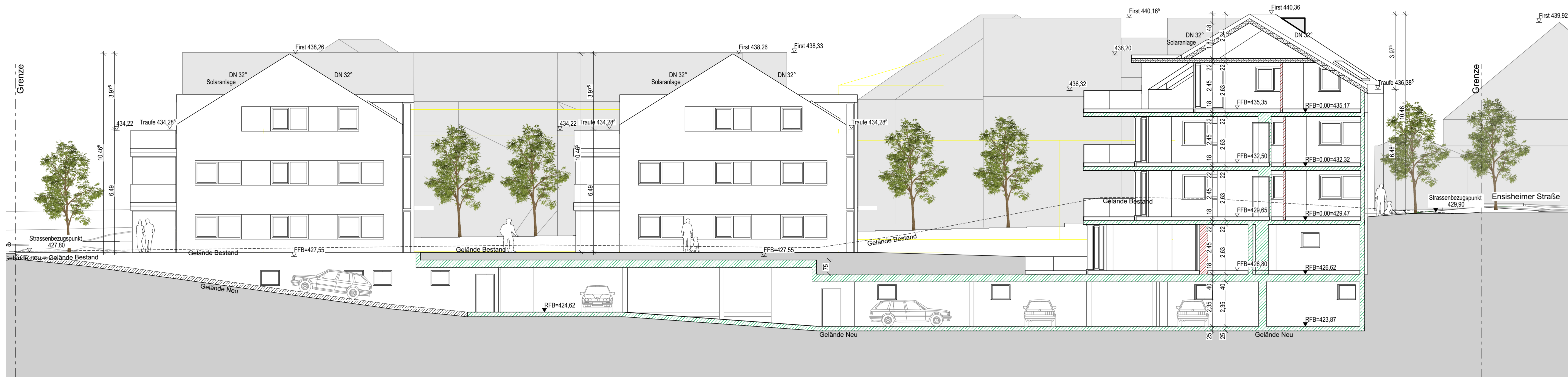
Schnitt A-A
