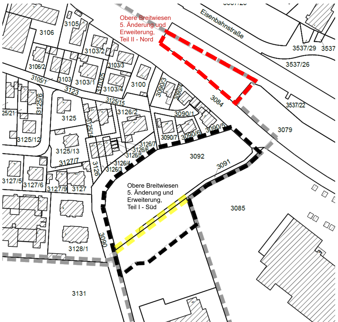
Abb. 2-2: Geltungsbereich des Bebauungsplans „Obere Breitwiesen 5. Änderung und Erweiterung, Teil I – Süd“ (schwarze Linie) sowie geplanter Geltungsbereich des Bebauungsplans „Obere Breitwiesen 5. Änderung und Erweiterung, Teil II – Nord“ (rote Linie)
