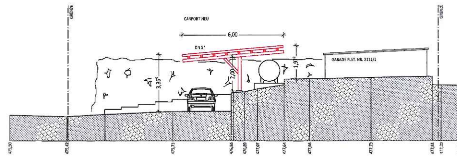
ANSICHT NORD/SCHNITT FLST. NR. 2112
