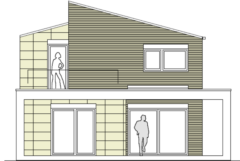
Ansicht West
