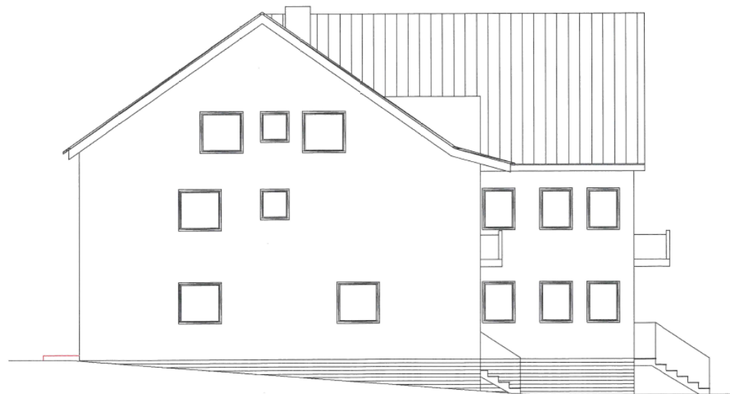
Ansicht West
