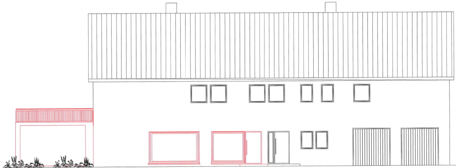
Ansicht Nord
