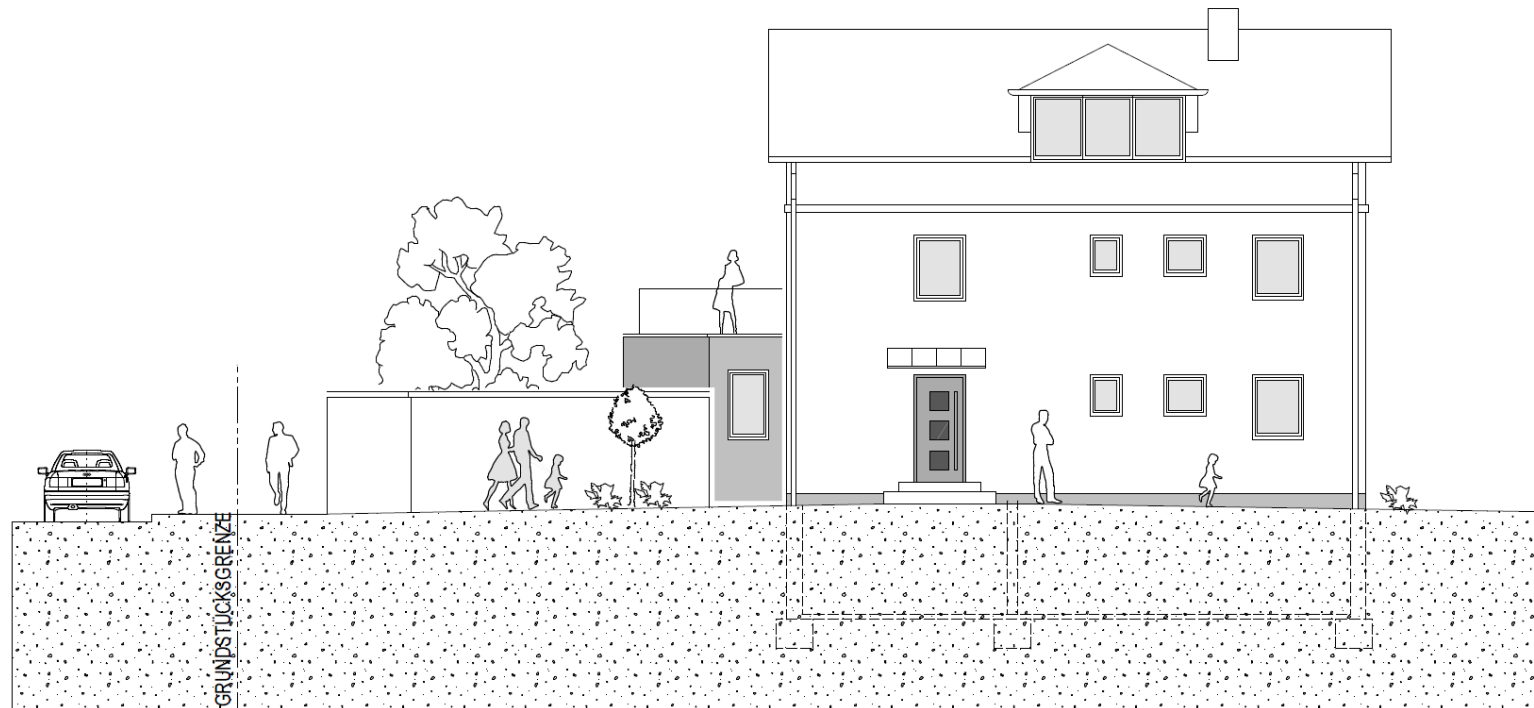
Ansicht Nord
