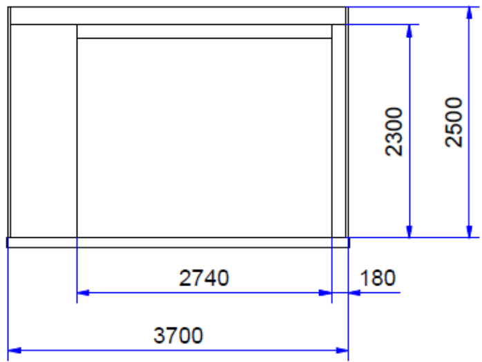
Ansicht Nod-Ost
