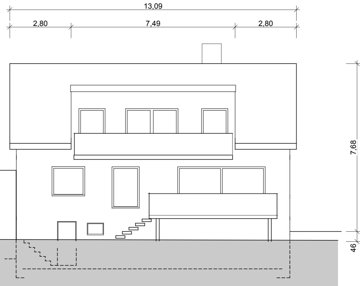
Ansicht Süd
