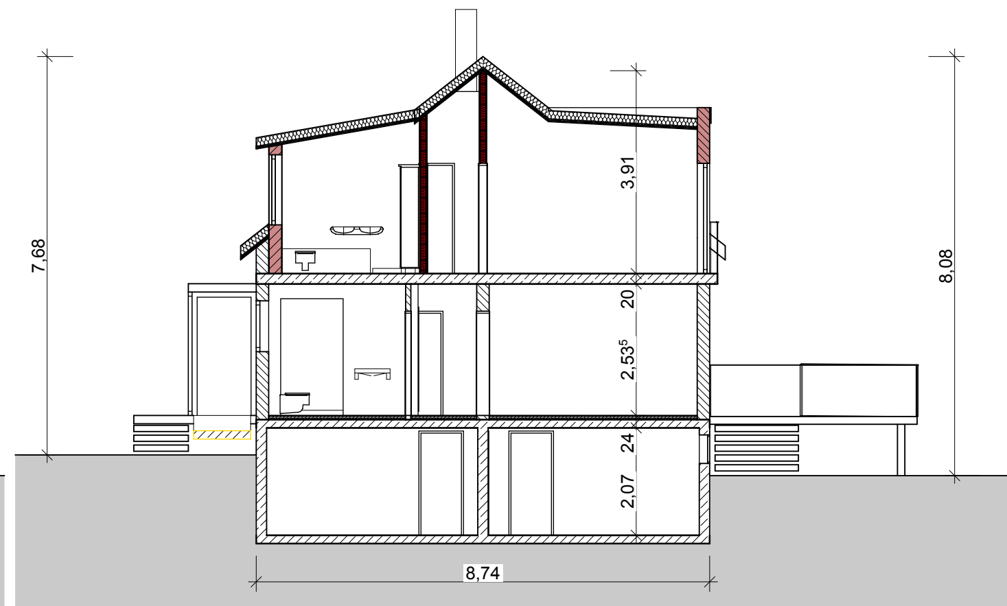
Schnitt 1
