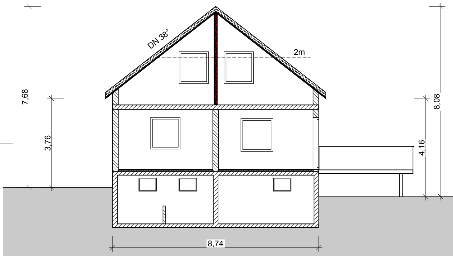
Schnitt 3
