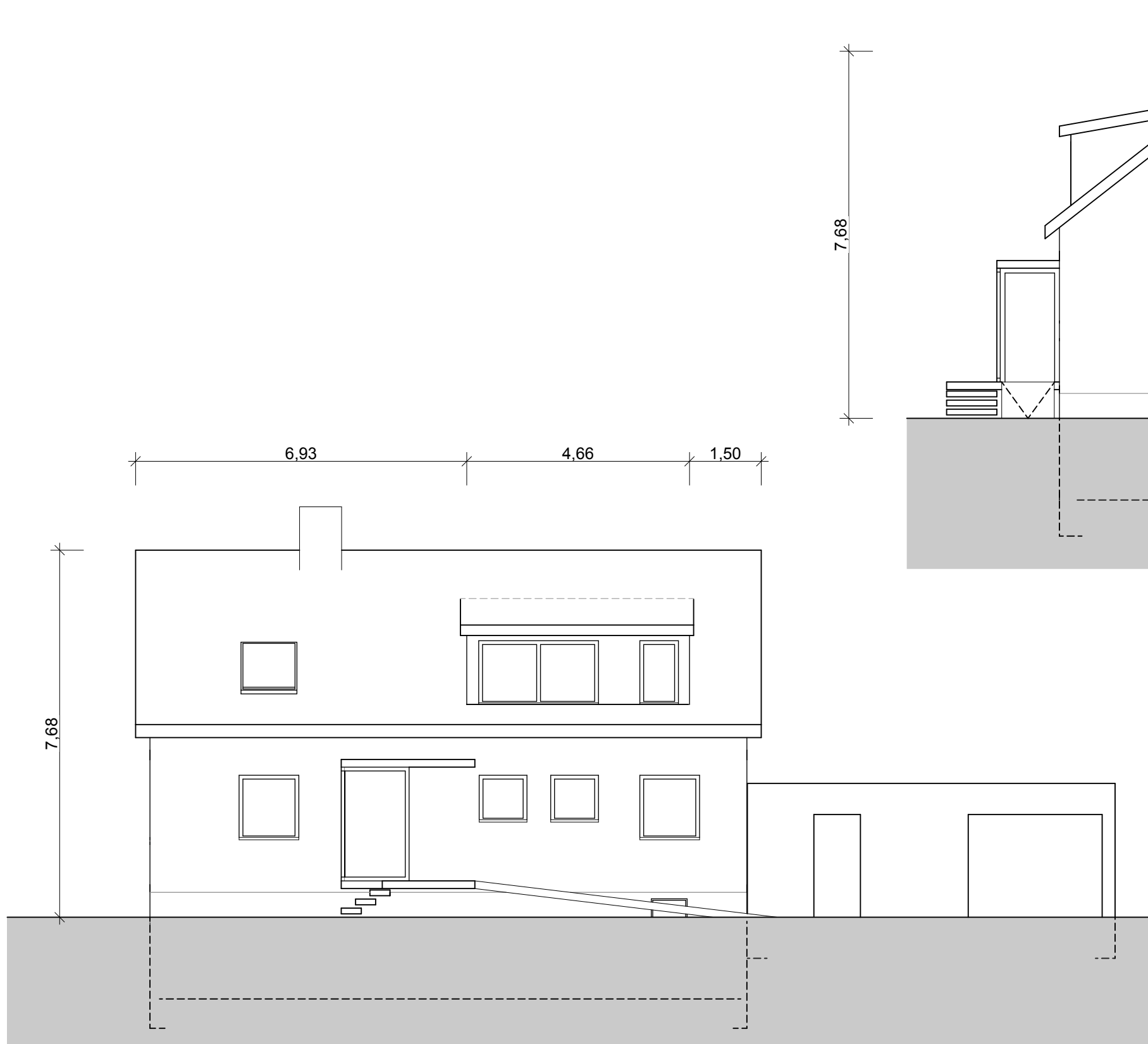
Ansicht Nord
