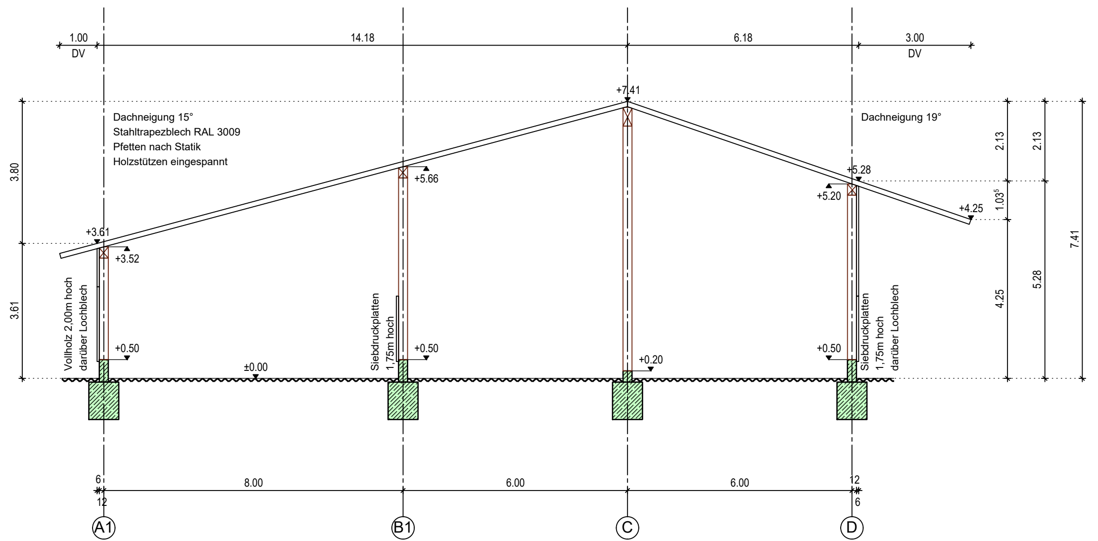
Schnitt B-B
