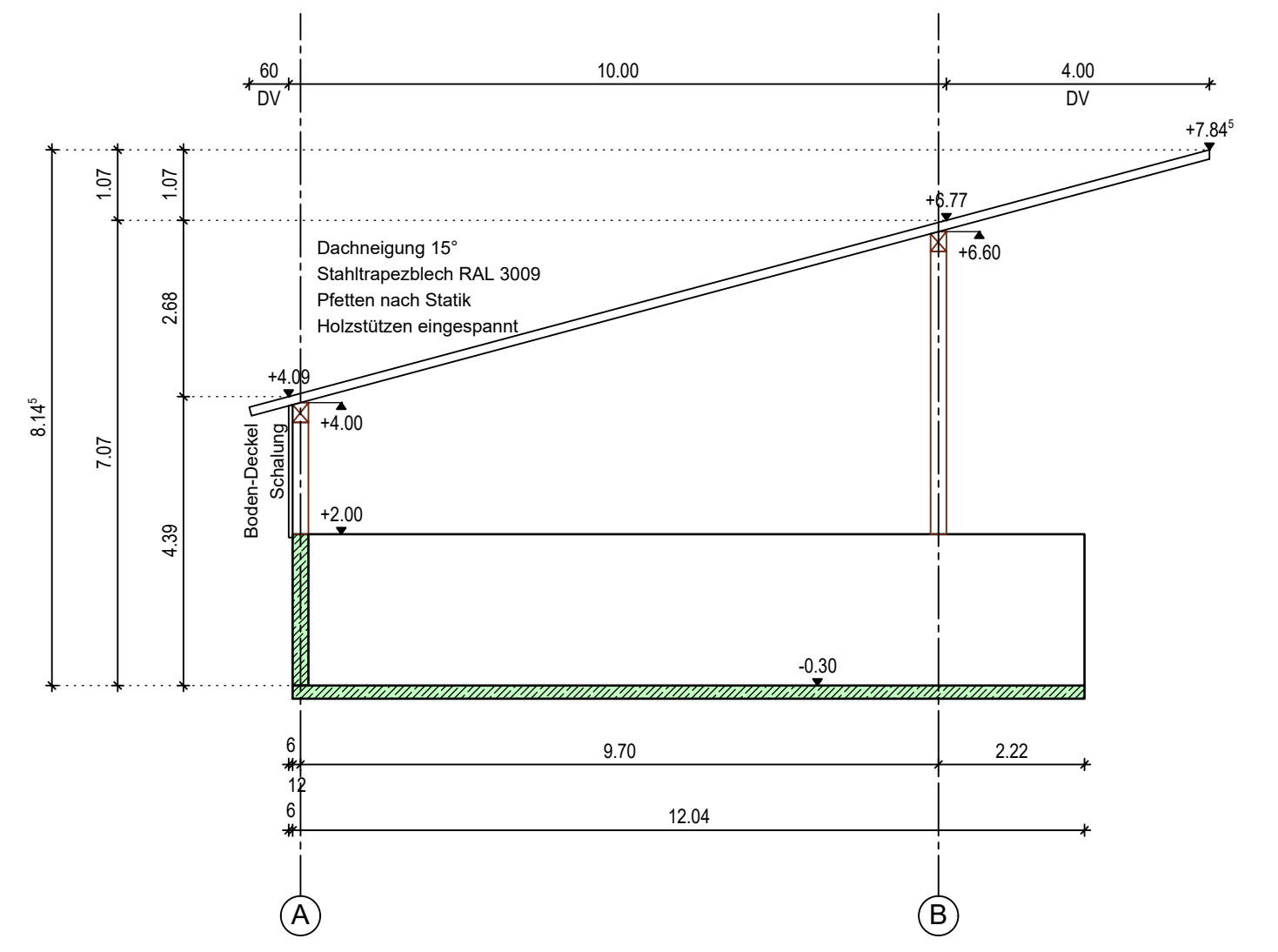
Schnitt C-C
