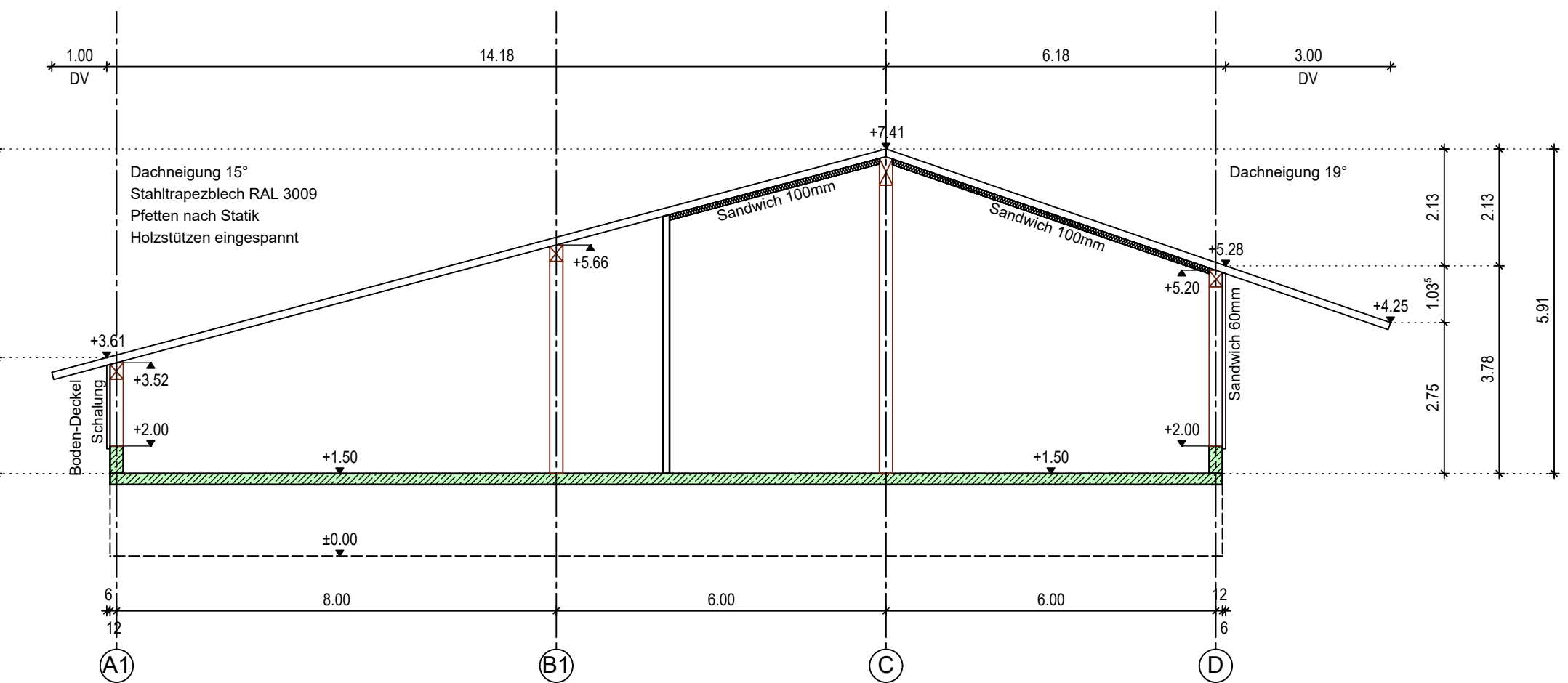
Schnitt A-A
