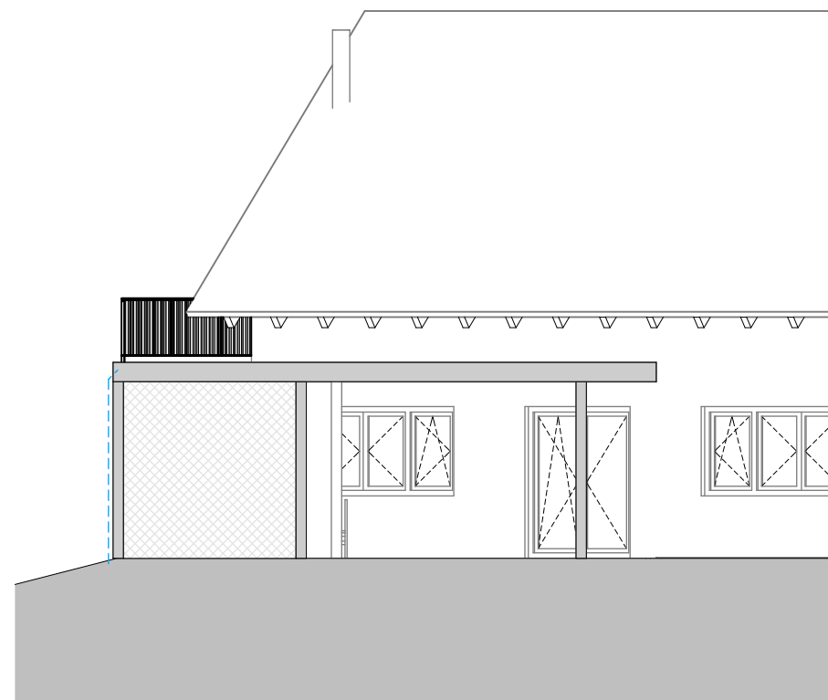
Ansicht Süd
