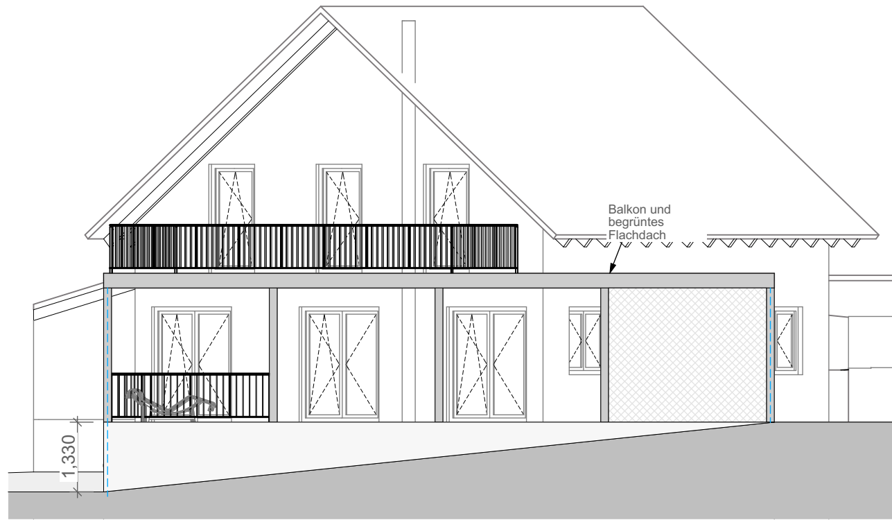
Ansicht West
