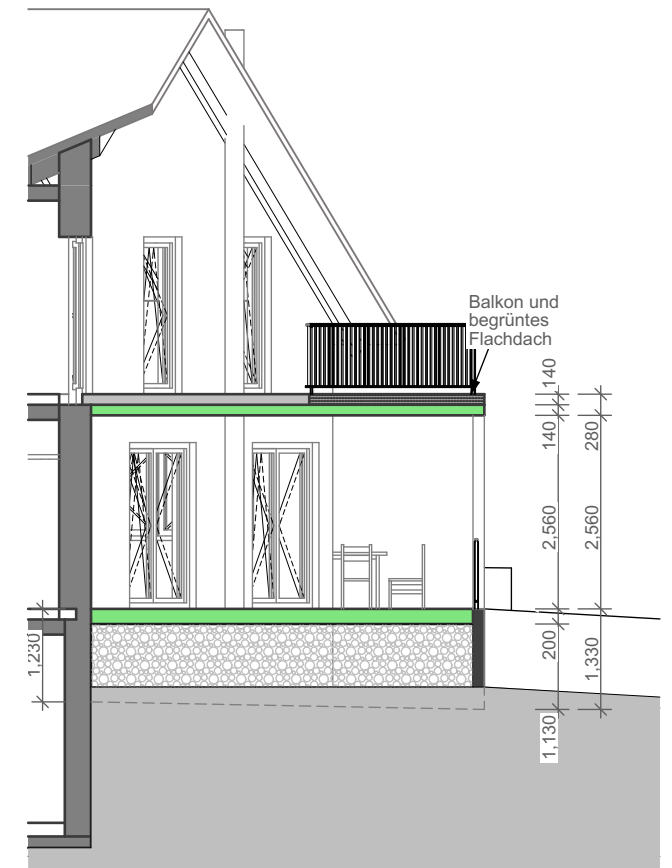
Schnitt
