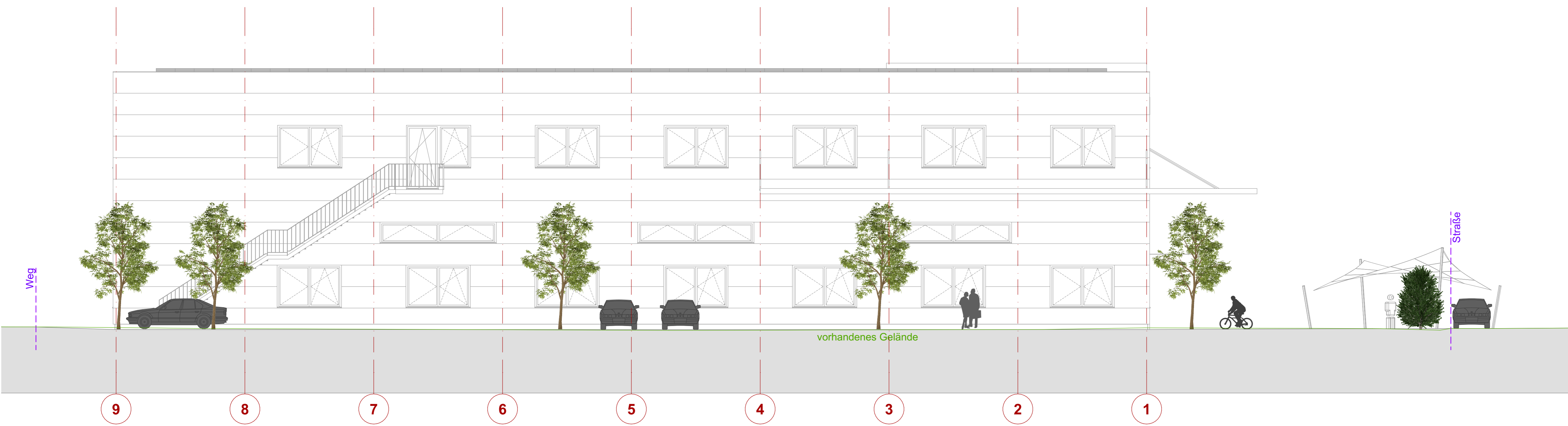
Ansicht NORD
