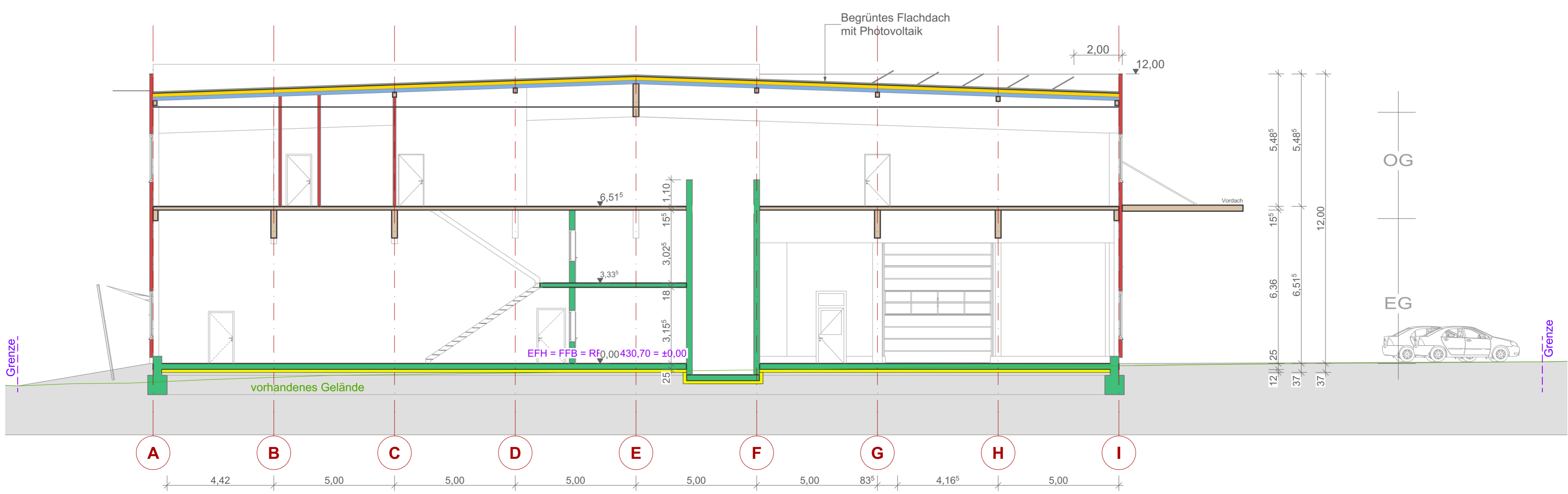
Schnitt B-B
