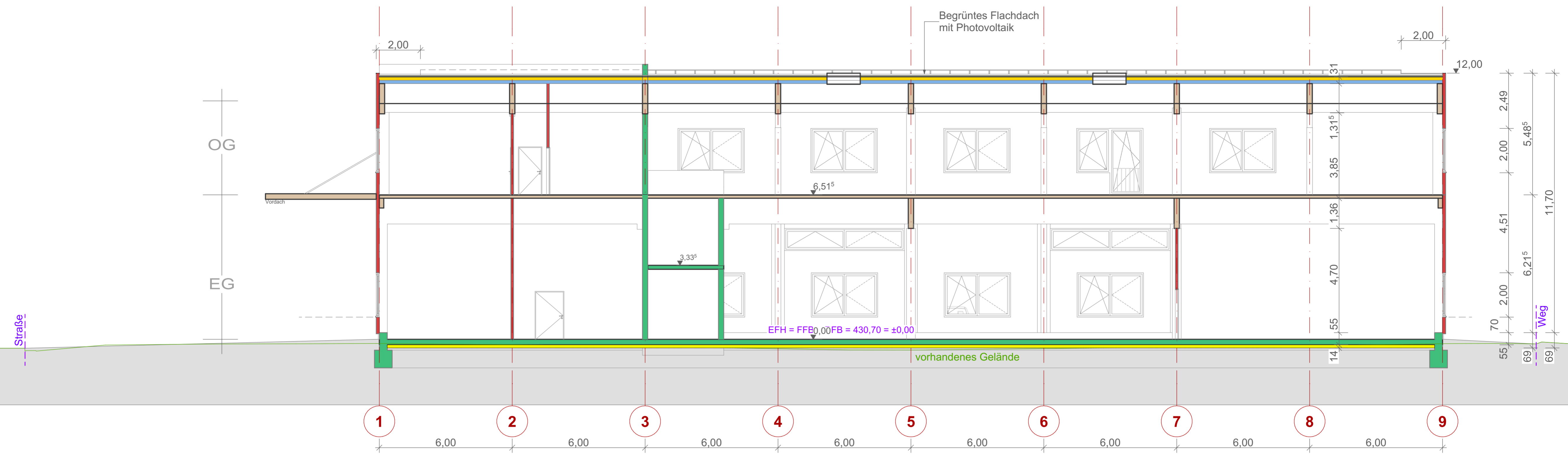
Schnitt A-A
